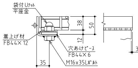
ボルト固定部詳細
