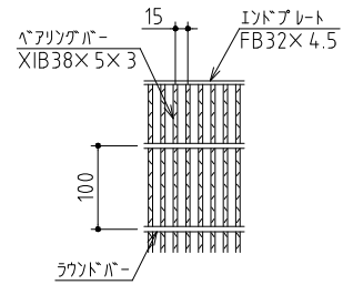
グレーチング構造図
